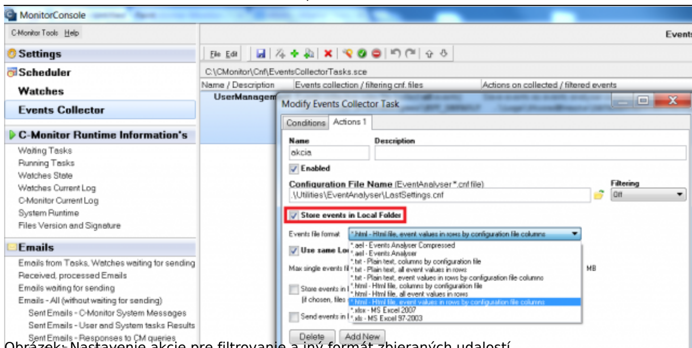
Obrázek: Nastavenie akcie pre filtrovanie a iný formát zbieraných udalostí
