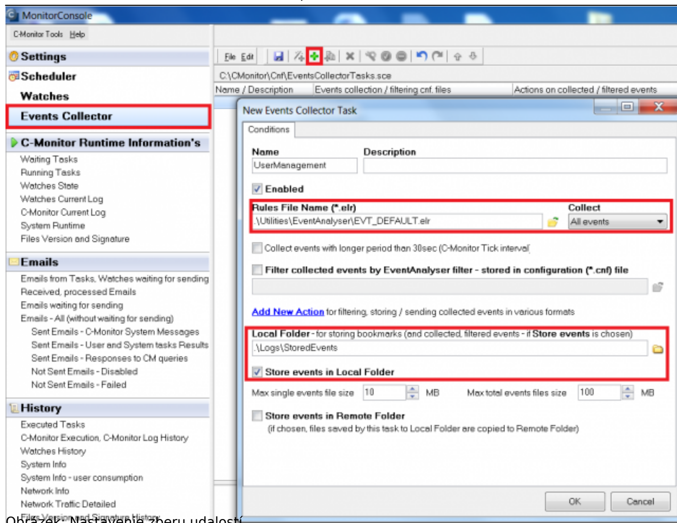
Obrazek: Nastavenie zberu udalostí
