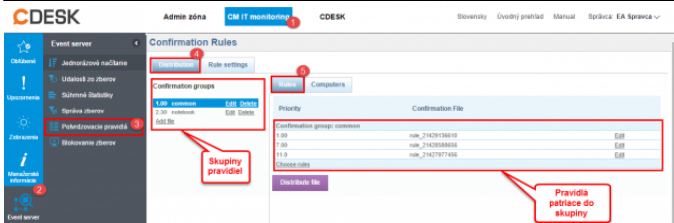
Obrázek: Zobrazenie a konfigurácia pravidiel potvrzovania
